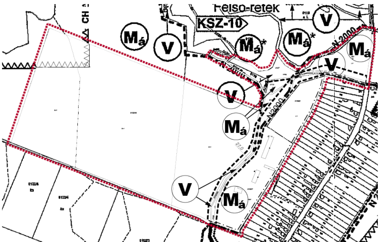
tervezett T-2 jelű külterületi szabályozási tervlap (részlet)
